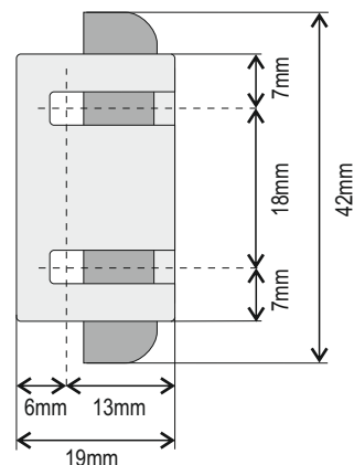
Detail bočního držáku roletky pohled ze spodu
