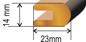
FEBA DOLNÍ PROFIL STANDARD
